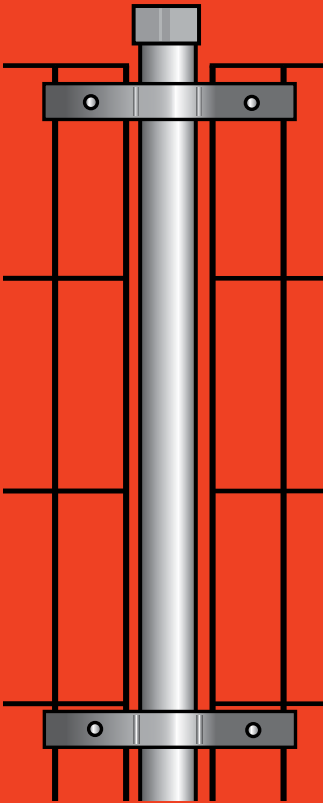
De bevestiging van de mat tussen de staander in detail
